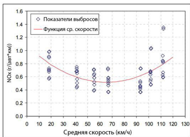
Рис. 1. Зависимость средней скорости от коэффициента выбросов [23]
