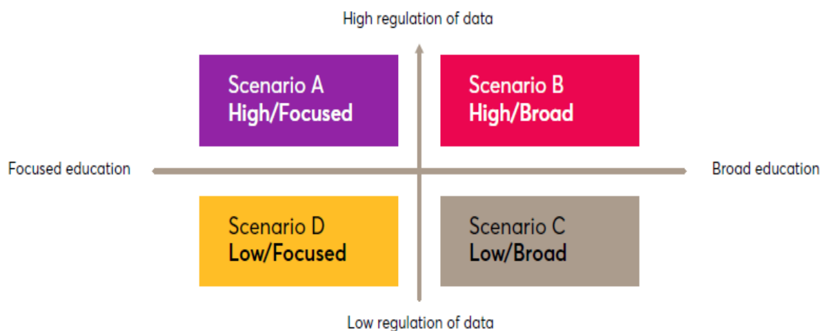
Рис. 2. Матрица сценариев
